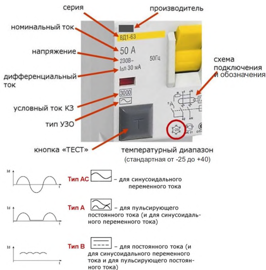
Рисунок 5. Маркировка УДТ
